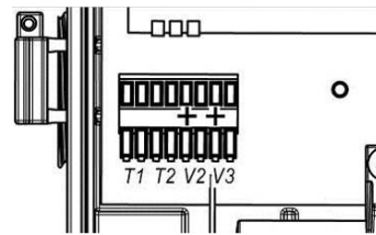
Расположение клемм «КСТ-22 КОМБИК-М РМД»
