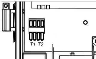
Расположение клемм «КСТ-22 КОМБИК-М»
